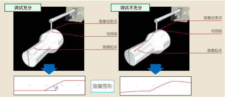
使用3轴调整工作台时的FORMTRACEPAK指导画面
