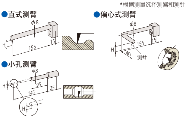
可应用测针列表(选件)
