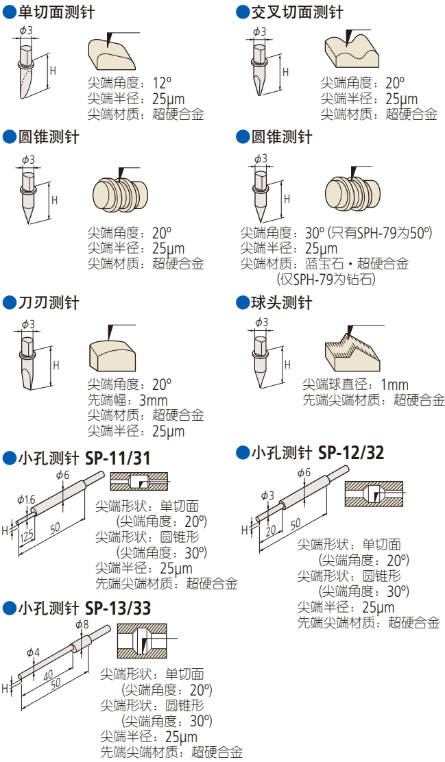
可应用测针列表(选件)
