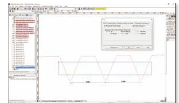
指定矩形螺纹间距范围的示例
